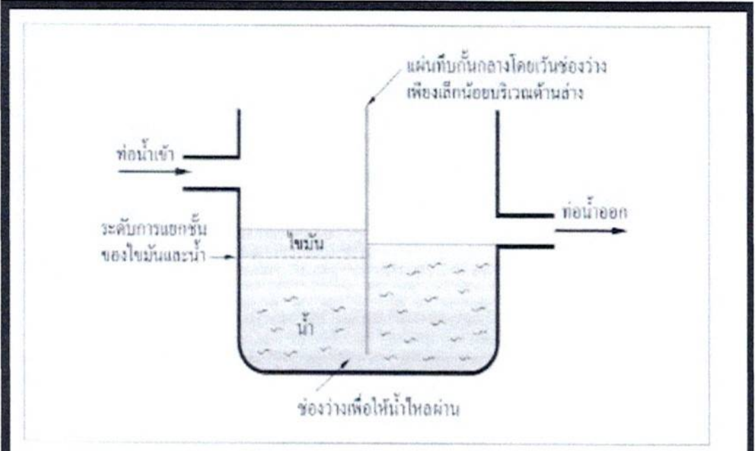
▲ ภาพแสดงระบบการทำงานแบบพื้นฐานของถังตกไขมัน
